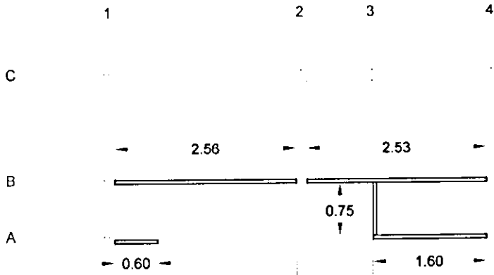
EDIFICIO B. PA MAMPARAS
